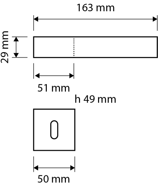
Технический чертёж, мм
