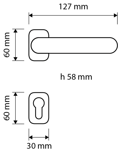
Технический чертёж, мм
